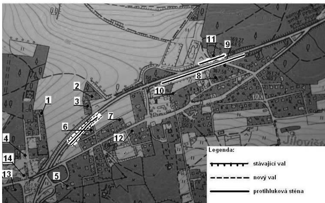
Protihluková opatření v obci Jíloviště se zakreslením měřených bodů
