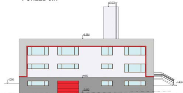
POHLED JIH
