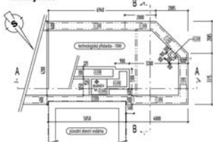
Základy...DSS
