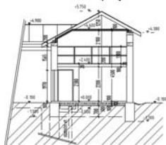
Řez příčný B-B...DSS
