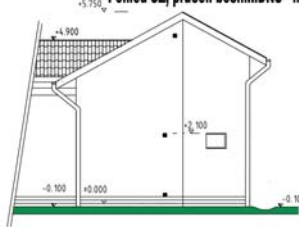
Pohled SZ, průčelí boční...DNS m 1:100
