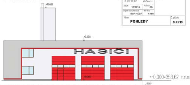
POHLED SEVER
