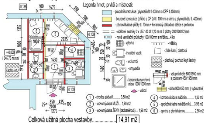
Pohled SV, průčelí vstupní...DNS m 1:100
