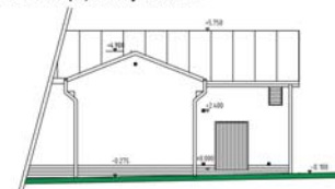
Pohled vstupní, severovýchodní...DSS
