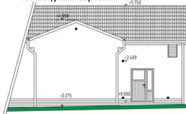
Pohled JZ, průčelí uliční...DNS m 1:100
