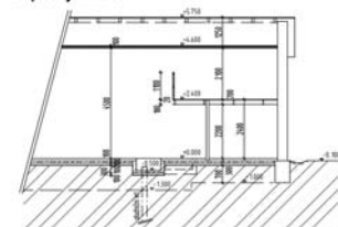
Řez podélný A-A...DSS
