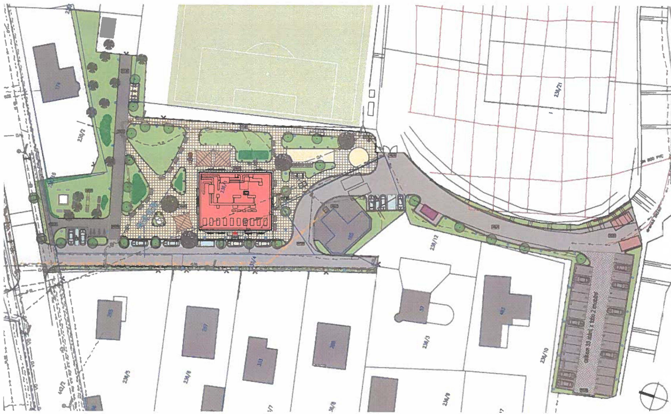
SITUACE - KOORDINAČNÍ - CELKOVÁ 1 : 500
